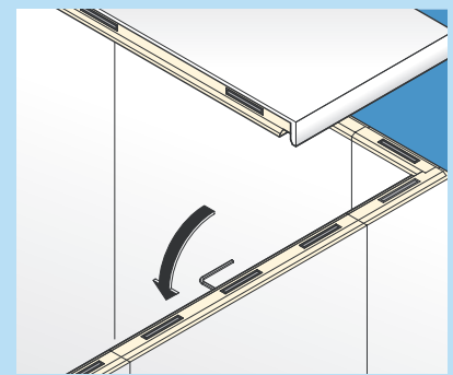
Deckenmontage
