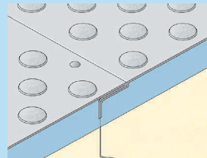
Edelstahlboden, kreisverpresst
