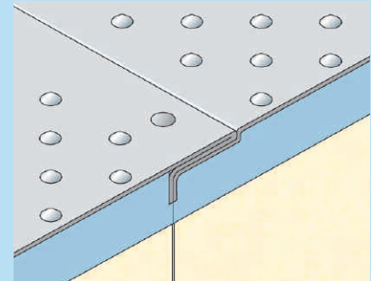
Edelstahlboden, kegelverpresst
